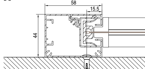
guida a parete - wall guide
