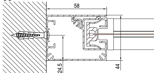
guida a nicchia - niche guide
